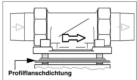
Abb. 3: Einbaudrehflansch
